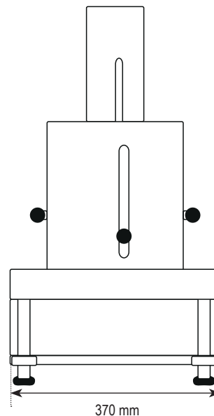
VUE DE FACE ■ FRONT VIEW ■ VOORAANZICHT
